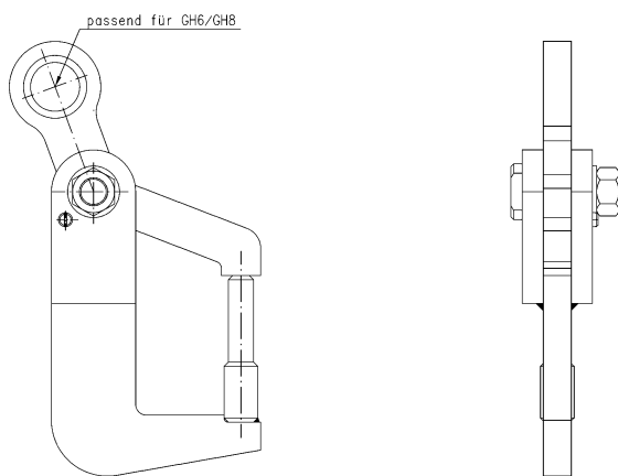
Darstellung Automatikhaken
